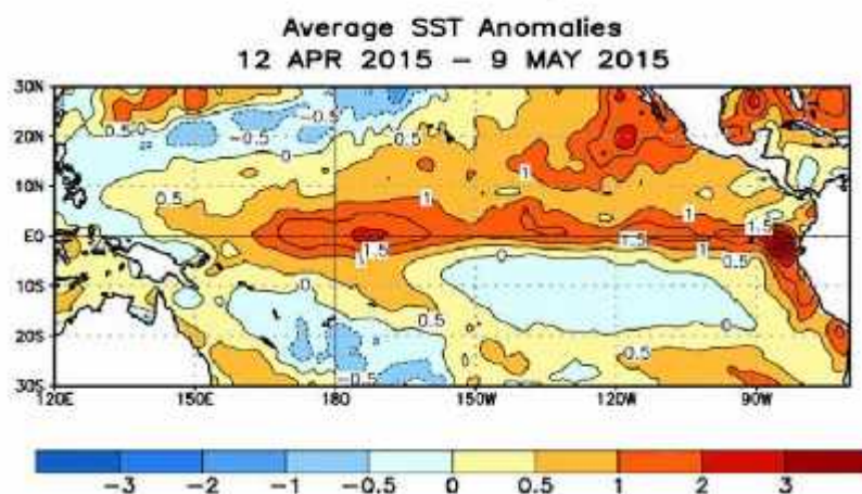
ภาพแสดงอุณหภูมิน้ำทะเลต่างจากค่าปกติ ระหว่างวันที่ 12 เมษายน - 9 พฤษภาคม 2558
